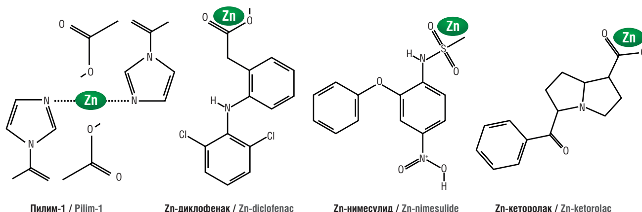
Рисунок 1. Химические формулы изученных молекул
