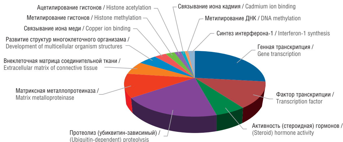
Рисунок 2. Анализ протеома и роль иона Zn^{2+} . Секторы диаграммы соответствуют количеству Zn^{2+} -зависимых белков по функционалу.
