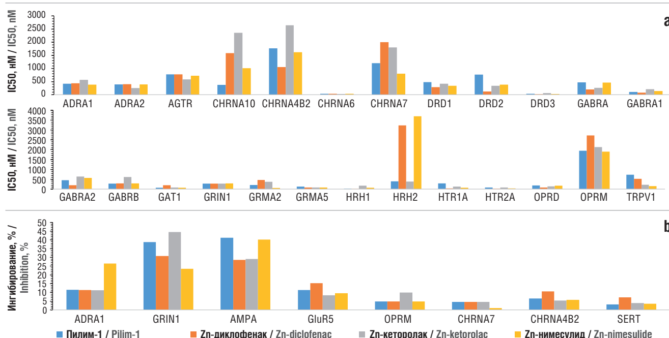
Рисунок 3. Хемореактомные оценки центральных эффектов пилима-1 и цинксодержащих нестероидных противовоспалительных препаратов:
